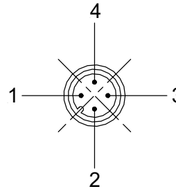
Steckeransicht am Sensor
